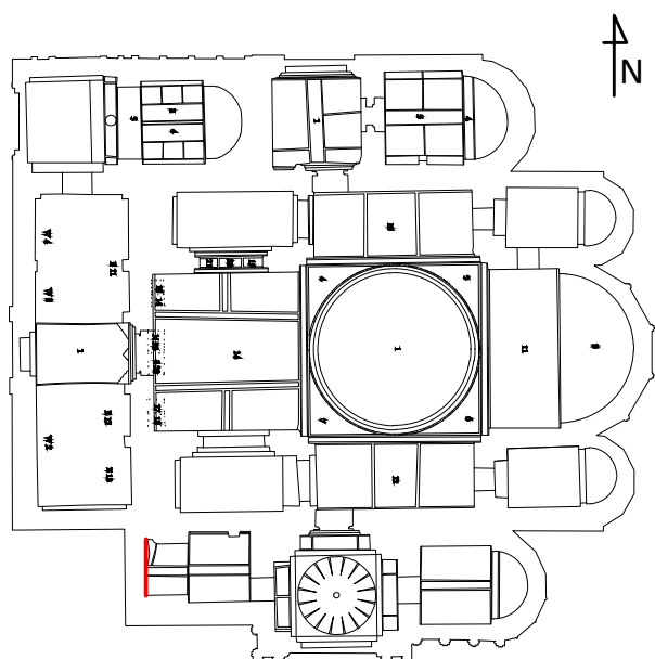
გეგმა / Plan
