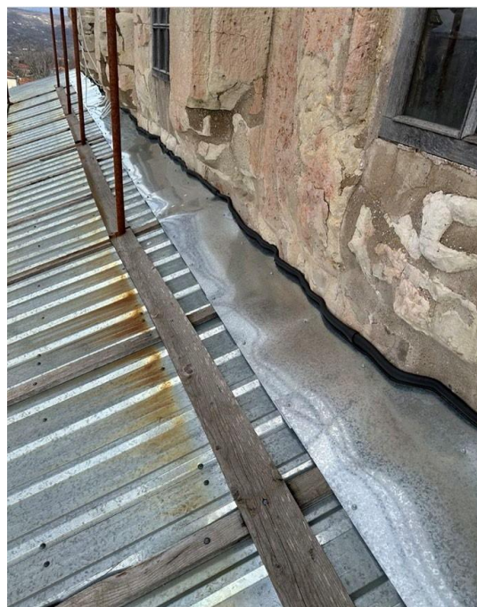
Fig. 15. დასავლეთ ფასადის ვერტიკალური კედლის - ნართექსის დროებით გადახურვასთან პრობლემური შეერთების ხაზი: ჩარევა შტორმის შემდეგ
