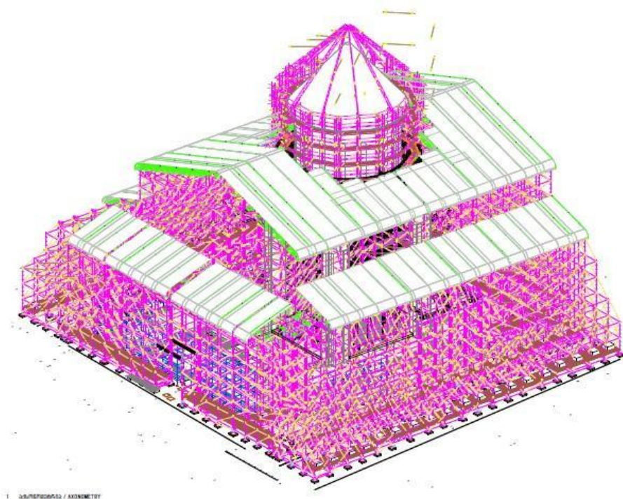
Fig. 2. მთავარი ტაძრის დროებითი გადახურვის კონსტრუქციული ნახაზი
