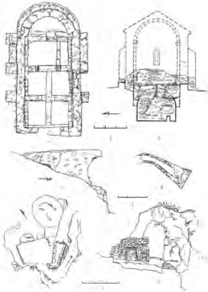
ტაბ. II. ღალიას ქართული მონასტერი. 1. წმ. ნიკოლოზის სახ. ეკლესია (ა. გეგმა, ბ. ჭრილი). 2. მონასტრის ნისქვილი (ა. აღმოსავლეთის ფასადი, ბ. ბე-ლლარის ზედახედი). 3. მარტომყოფელი ბერის სენაკი (ა. გეგმა, ბ. ჭრილი).
