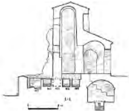
ნეკრესის აკლდამები და ჭრილი
